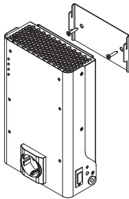
Рисунок 10а Крепление стабилизаторов Штиль ИнСтаб IS350 и IS550 на ровной вертикальной поверхности
