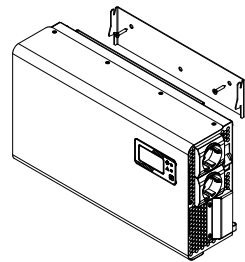
Рисунок 10в Крепление стабилизаторов Штиль ИнСтаб IS2500 и IS3500 на ровной вертикальной поверхности
