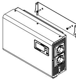
Рисунок 10б Крепление стабилизаторов Штиль ИнСтаб IS1000 и IS1500 на ровной вертикальной поверхности
