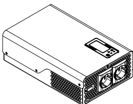
Рисунок 11а Горизонтальная установка стабилизаторов Штиль ИнСтаб IS1000 и IS1500
