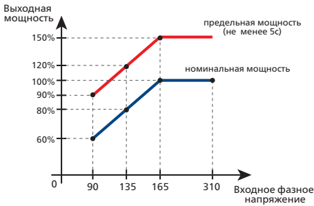
Рисунок 9 Зависимость выходной мощности от входного напряжения
